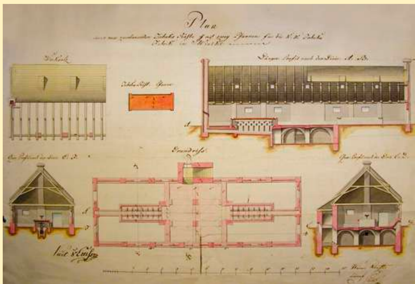
ПЛАН РОЗШИРЕННЯ БУДИНКУ ДЛЯ СУШІННЯ ТЮТЮНУ В С.ВИННИКИ,1818 р. ЦДІАЛ.- Ф.726, оп.1, спр.669 PLAN OF THE ENLARGEMENT OF THE BUILDING FOR DRYING TOBACCO IN VILLAGE VYNNYKY, 1818. CSHAL. - Fund 726, Description 1, Case 669
