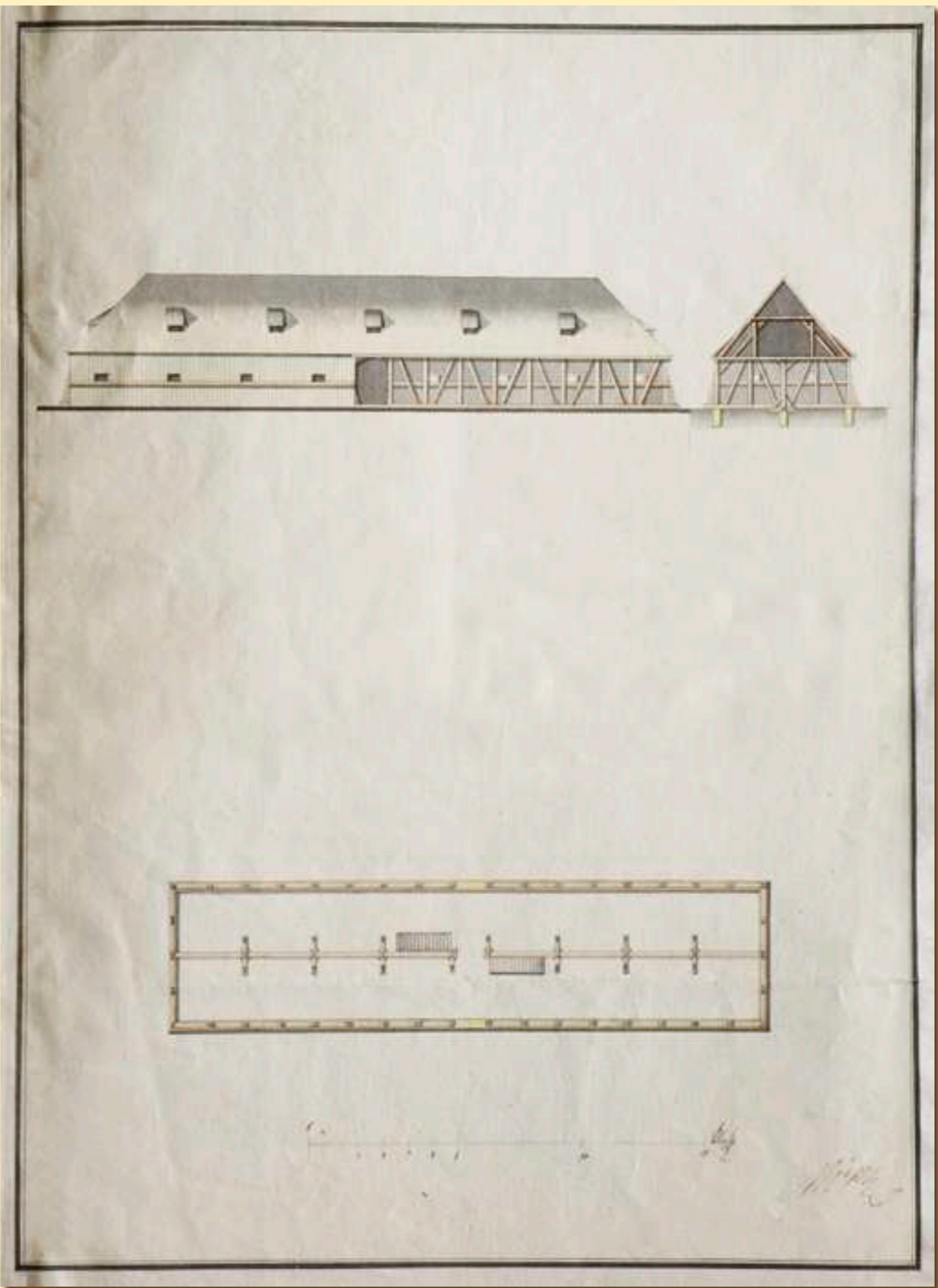
ПЛАН БУДІВЛІ СКЛАДУ ТЮТЮНУ, 1784 р. ЦДІАЛ. - Ф.726, оп.1, спр.652 DRAFT OF THE BUILDING FOR A TOBACCO WAREHOUSE, 1784. CSHAL. - Fund 726, Description 1, Case 652
