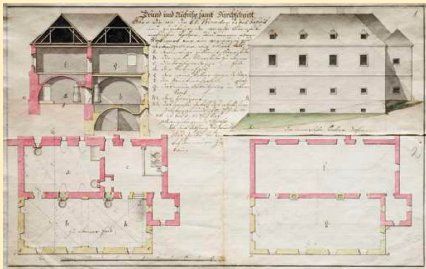
ПЛАН БУДІВНИЦТВА ПРИМІЩЕНЬ ДЛЯ СУШІННЯ ТЮТЮНУ, 1793 р. ЦДІАЛ. - Ф.726, он.1, спр.653 CONSTRUCTION DRAFT OF BUILDINGS FOR DRYING TOBACCO, 1793. CSHAL. - Fund 726, Description 1, Case 653
