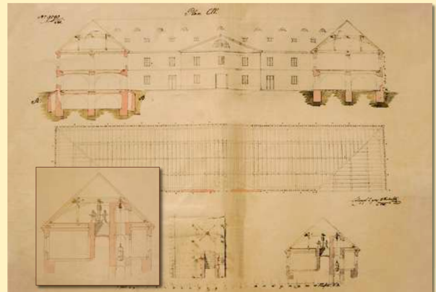
ПЛАН РОЗБУДОВИ СХІДНОЇ ТА ПІВДЕННОЇ ЧАСТИНИ БУДИНКУ ТЮТЮНОВОЇ ФАБРИКИ В С. ВИННИКИ, 1840 р. ЦДІАЛ.- Ф.726, оп.1, спр.685 ENLARGEMENT PLAN OF THE EASTERN AND SOUTHERN PARTS OF THE TOBACCO FACTORY'S BUILDING IN VILLAGE VYNNYKY, 1840. CSHAL. - Fund 726, Description 1, Case 685
