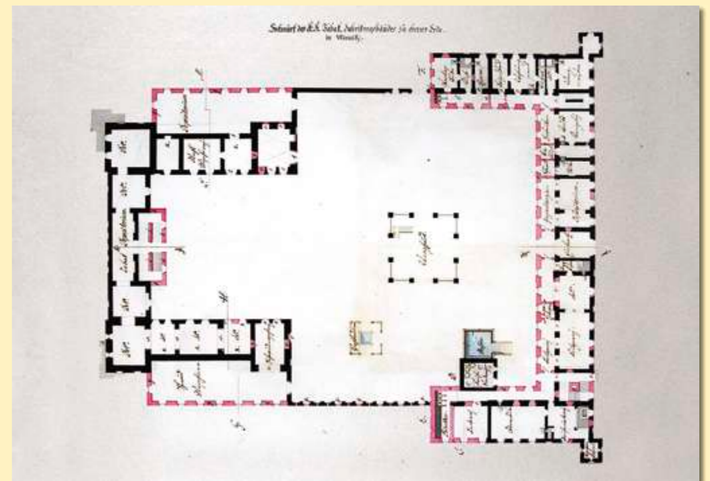
ПЛАН ПЕРЕБУДОВИ ПРИМІЩЕНЬ ЗАМКУ В ТЮТЮНОВУ ФАБРИКУ, 1796 р. ЦДІАЛ. - Ф.726, он.1, спр.654 PLAN OF THE RECONSTRUCTION OF THE CASTLE PREMISES INTO THE TOBACCO FACTORY, 1796. CSHAL. - Fund 726, Description 1, Case 654
