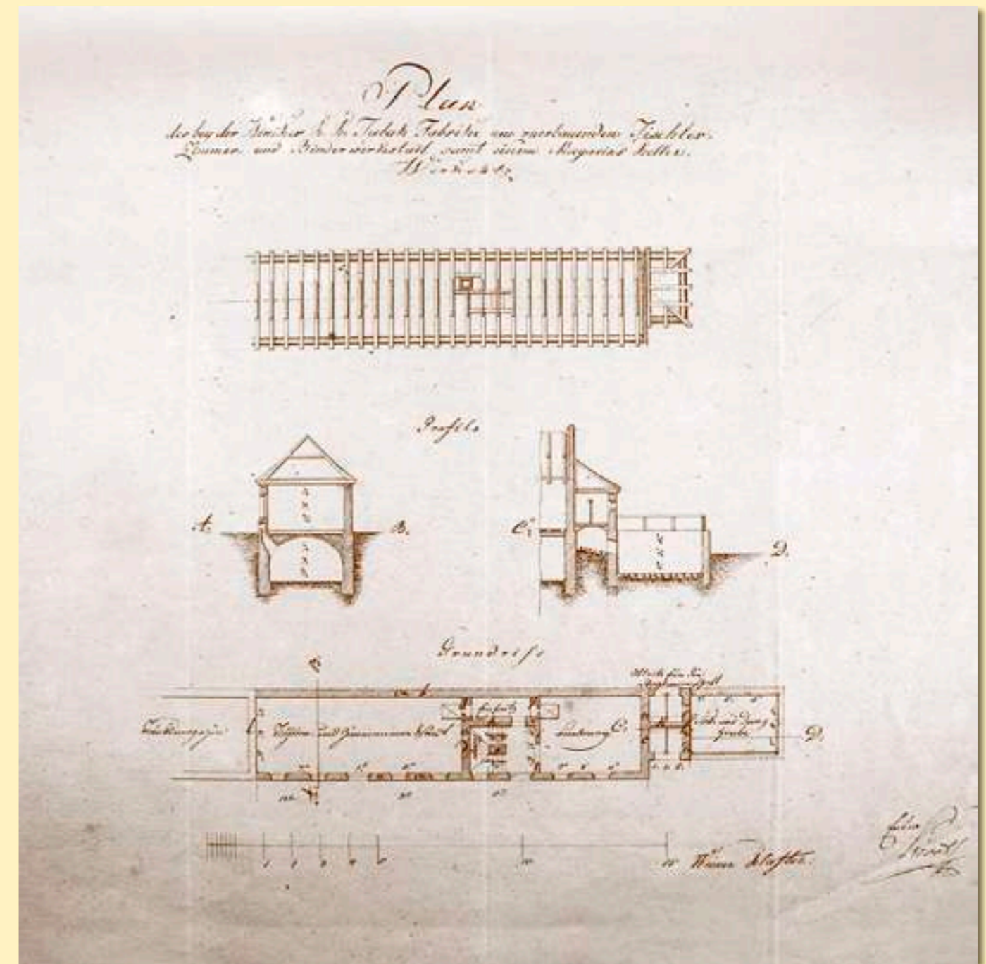
ПЛАН БУДОВИ СТОЛЯРНІ ТА БОНДАРСЬКОЇ МАЙСТЕРНІ ТЮТЮНОВОЇ ФАБРИКИ, 1818 р. ЦДІАЛ. - Ф.726, on.1, спр.663 RECONSTRUCTION PLAN OF THE TOBACCO FACTORY'S JOINER'S AND COOPER'S SHOPS, 1818. CSHAL. - Fund 726, Description 1, Case 663
