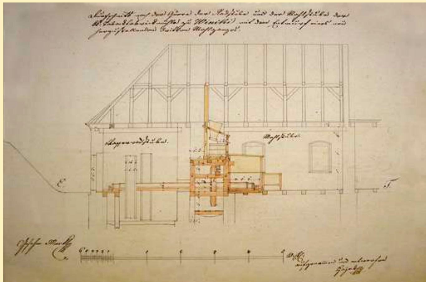
ПЛАН БУДІВНИЦТВА МЛИНА ТЮТЮНОВОЇ ФАБРИКИ У С. ВИННИКАХ НА Р. МАРУНЬКА, 1799 Р. ЦДІАЛ. - Ф.726, оп.1, спр.655 DRAFT OF THE CONSTRUCTION OF THE TOBACCO FACTORY'S WATERMILL IN VILLAGE VYNNYKY ON THE MARUN'KA RIVER, 1799. CSHAL. - Fund 726, Description 1, Case 655
