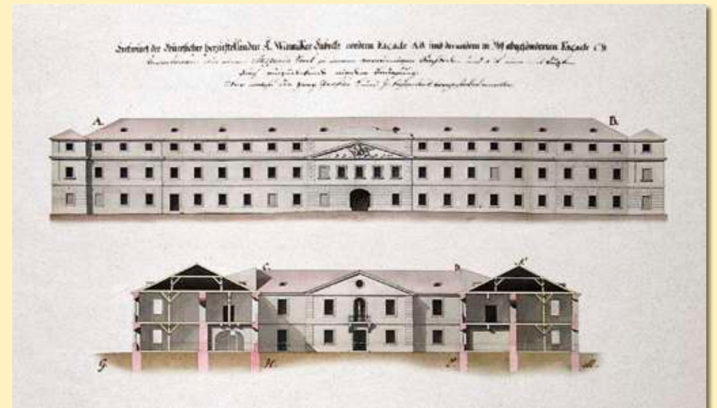
ПЛАН БУДІВЛІ ТЮТЮНОВОЇ ФАБРИКИ, 1797 р. ЦДІАЛ. - Ф.726, он.1, спр.654 DRAFT OF THE TOBACCO FACTORY BUILDING, 1797. CSHAL. - Fund 726, Description 1, Case 654
