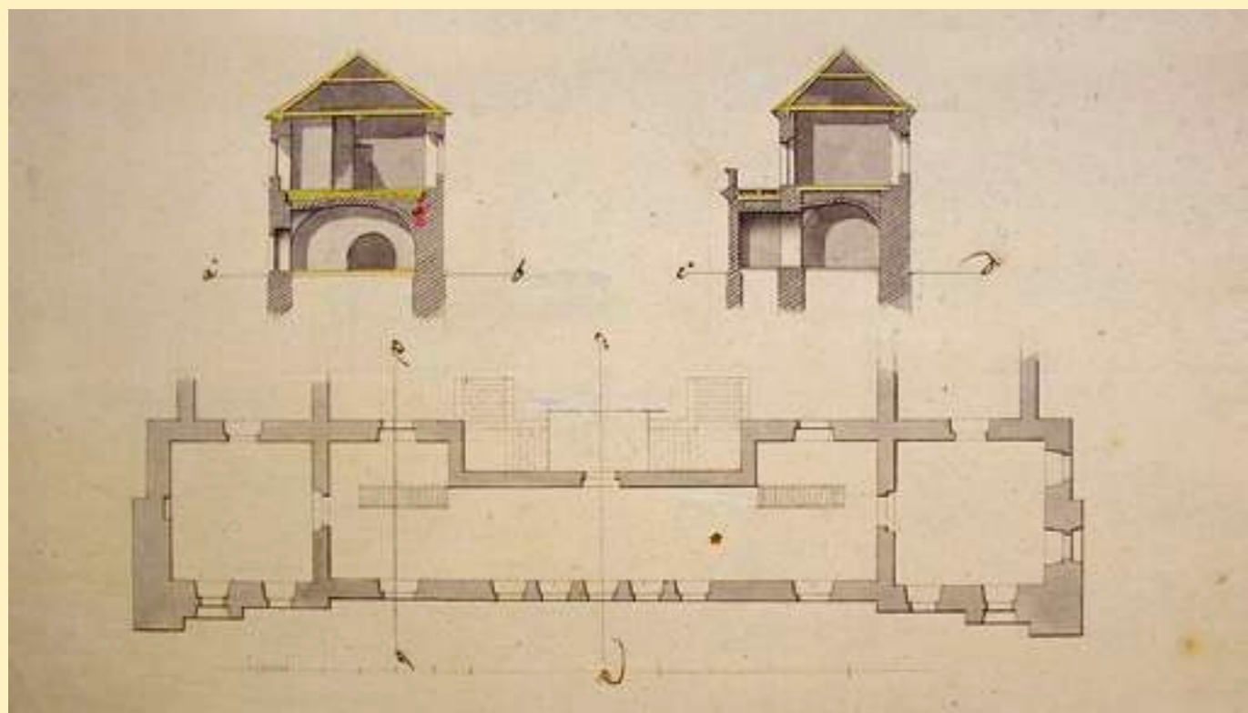
ПЛАН ПРИМІЩЕНЬ ГОСПОДАРСЬКОГО СКЛАДУ ТЮТЮНОВОЇ ФАБРИКИ В С. ВИННИКИ, 1818 р. ЦДІАЛ.- Ф.726, оп.1, спр.667 PLAN OF THE HOUSEHOLD WAREHOUSE'S BUILDINGS OF THE TOBACCO FACTORY IN VILLAGE VYNNYKY, 1818. CSHAL. - Fund 726, Description 1, Case 667
