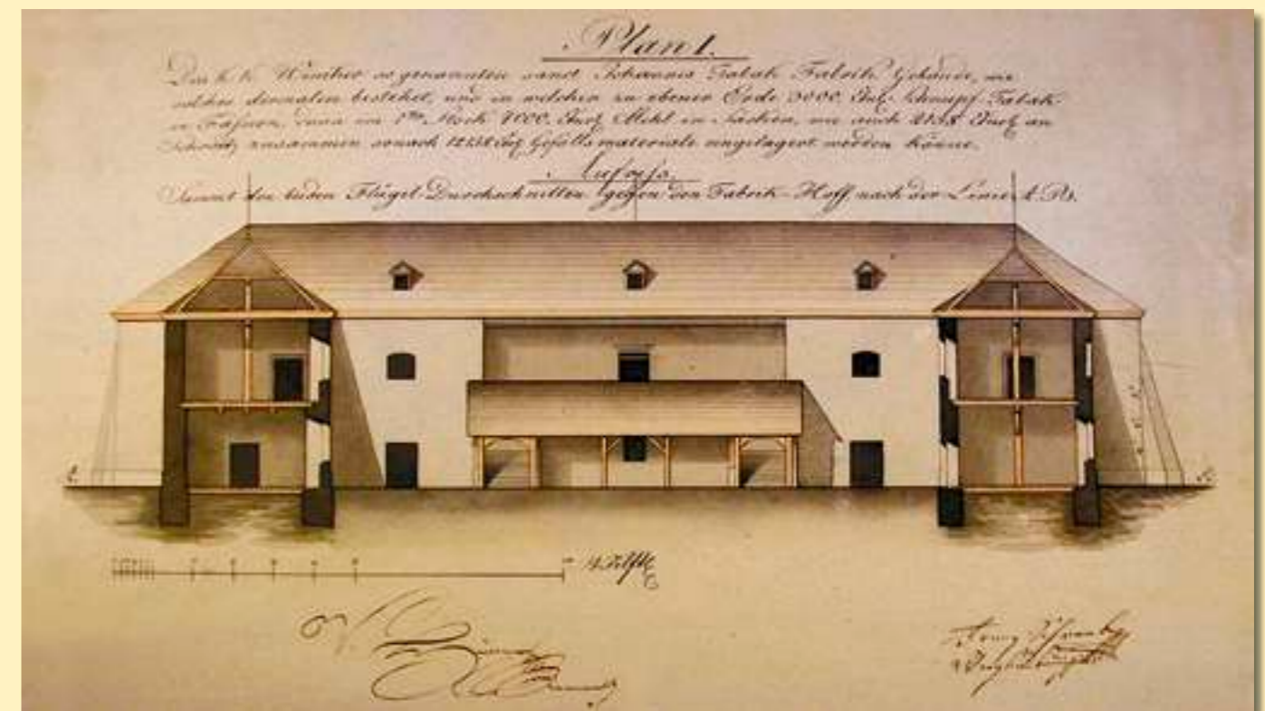
ПЛАН БУДІВЛІ ТЮТЮНОВОЇ ФАБРИКИ В С. ВИННИКИ, 1882 р. ЦДІАЛ.- Ф.726, оп.1, спр.679 PLAN OF THE TOBACCO FACTORY'S BUILDING IN VILLAGE VYNNYKY, 1882. CSHAL. - Fund 726, Description 1, Case 679
